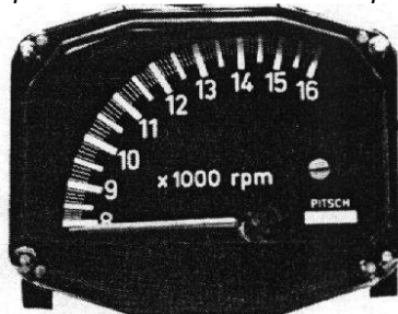
Modello speciale 8000 - 16000 giri al minuto Special model 8000 - 16000 rpm
