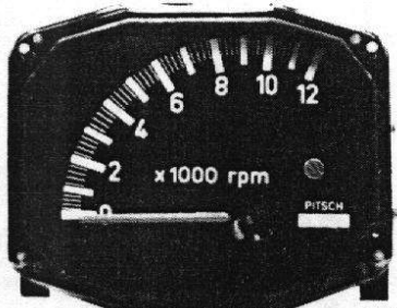
Modello standard 0 - 12000 giri al minuto Standard model 0 - 12000 rpm
