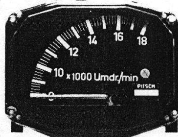
Modello speciale 8000 - 18000 giri al minuto Special model 8000 - 18000 rpm
